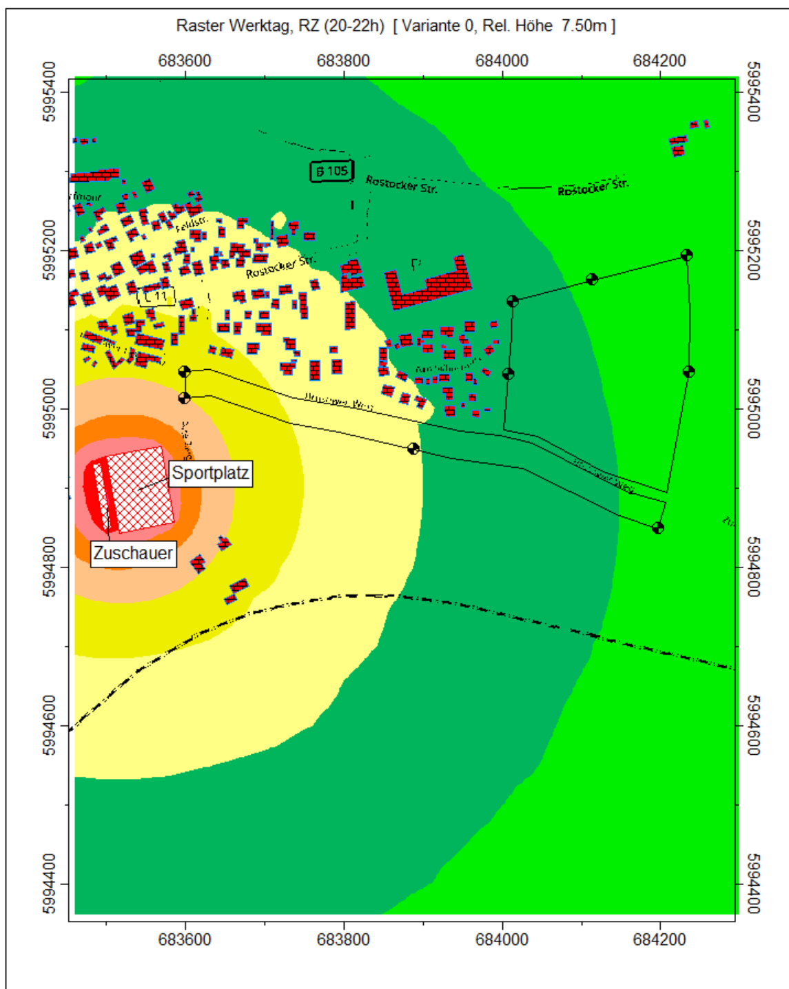
Abbildung 16: Rasterlärmkarte Sportanlage Werktag 20-22 Uhr (UTM-Koordinaten)
