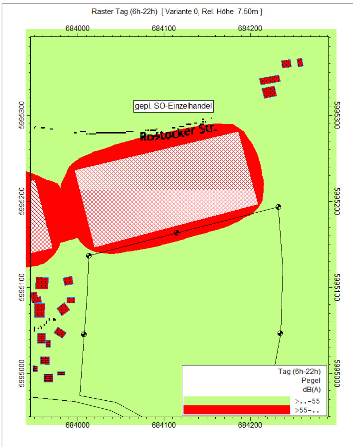
Abbildung 8: Ausschnitt Überschreitungen - Rasterlärmappe Gewerbe Werktag 06-22 Uhr (UTM-Koordinaten)
