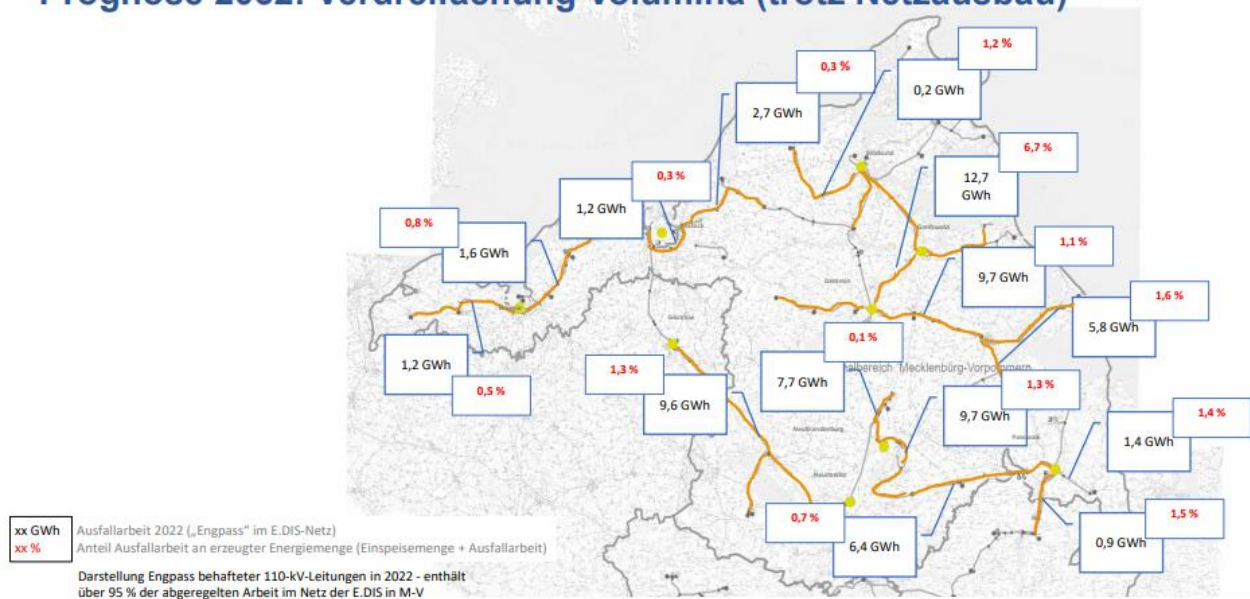
Abbildung 67: Trassenbezogene Abregelmengen in 2022 (Quelle: Montebaur 2023) 38
