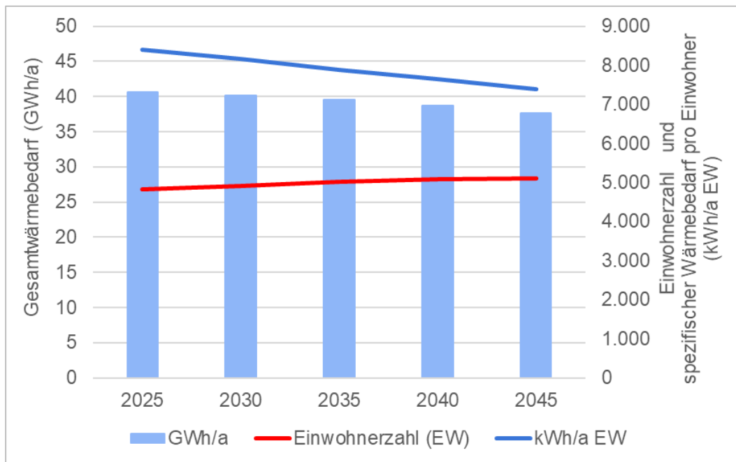
Abbildung 32: Erwartete Wärmebedarfsentwicklung gesamt und pro Einwohner in Kröpelin
