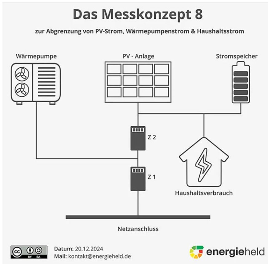
Abbildung 48: Kaskadenschaltung für eine optimierte Stromnutzung (Quelle: Energieheld)
