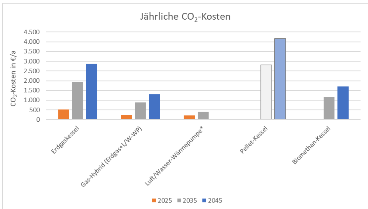
Abbildung 52: CO 2 -Kosten der Wärmeversorgung im EFH Beispiel 1
