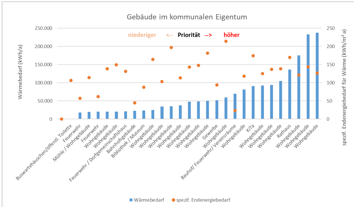
Abbildung 31: Wärmebedarf, spezifischer Wärme- und Endenergiebedarf der kommunalen Liegenschaften (Quelle: LGMV, eigene Auswertung)
