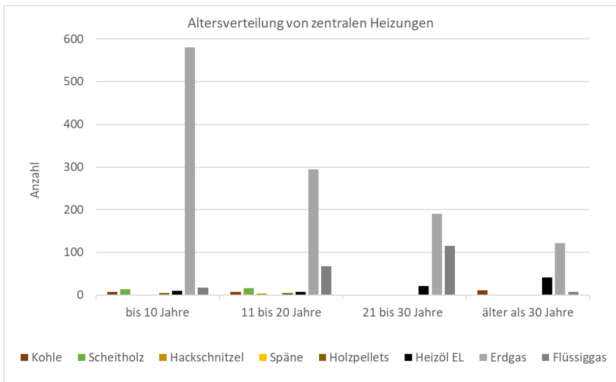
Abbildung 23: Altersverteilung der zentralen Heizungen nach Brennstoff (Quelle: eigene Auswertung von Kehr- buchdaten)
