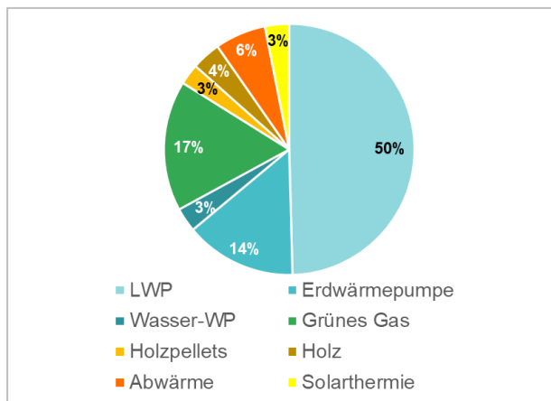
Abbildung 39: Anteile der Heizsysteme inkl. der zentralen Wärmeversorgung im Zielszenario 2045
