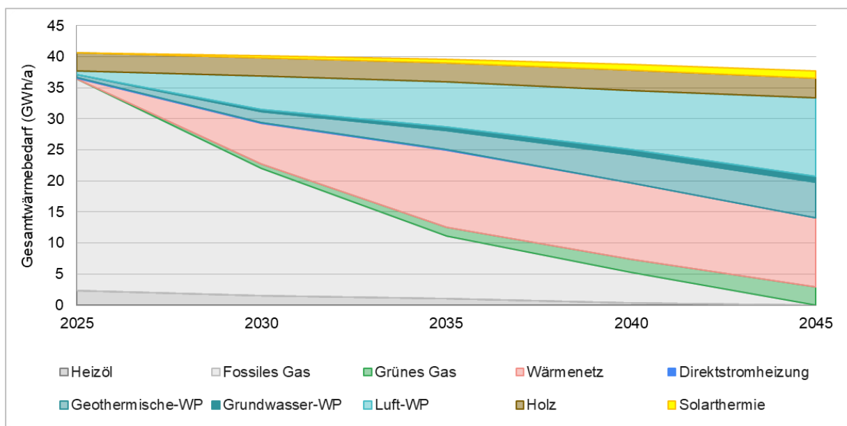
Abbildung 40: Szenario zum Gesamtwärmebedarf nach Energieträger (urbio)
