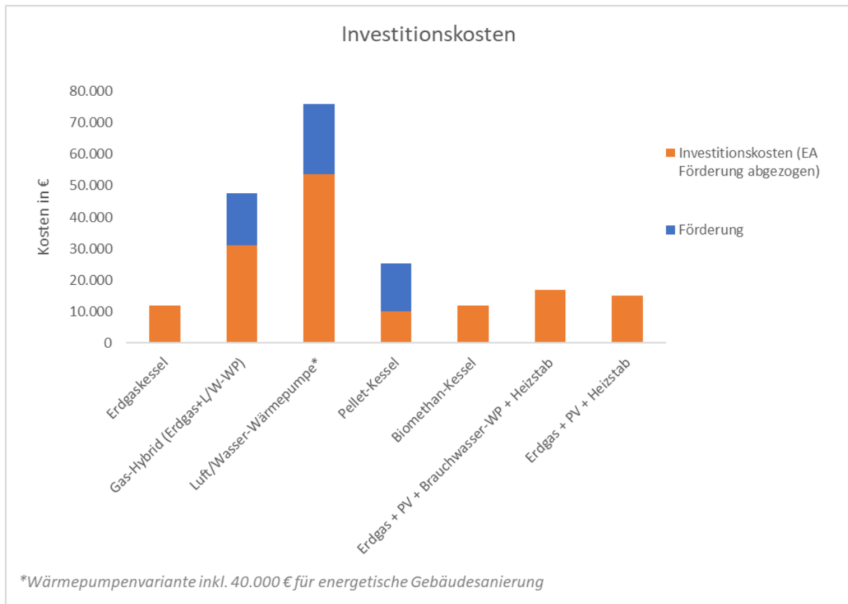
Abbildung 50: Investitionskosten EFH Beispiel 1
